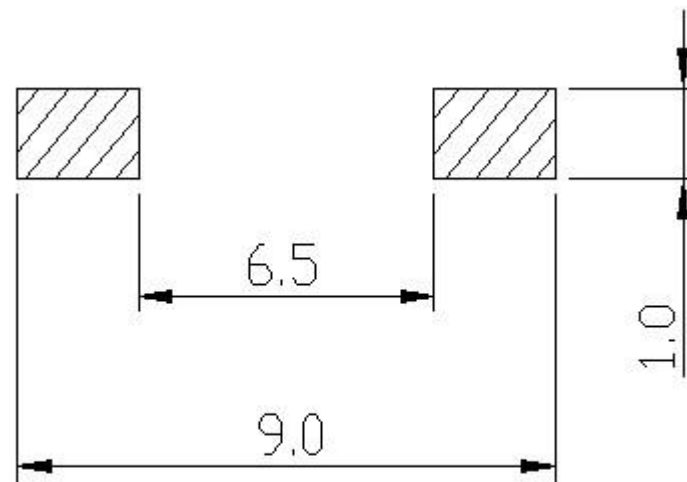
P.C.B LAND DIMENSION
