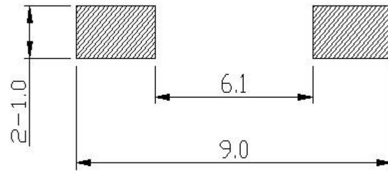
P.C.B LAND DIMENSION
