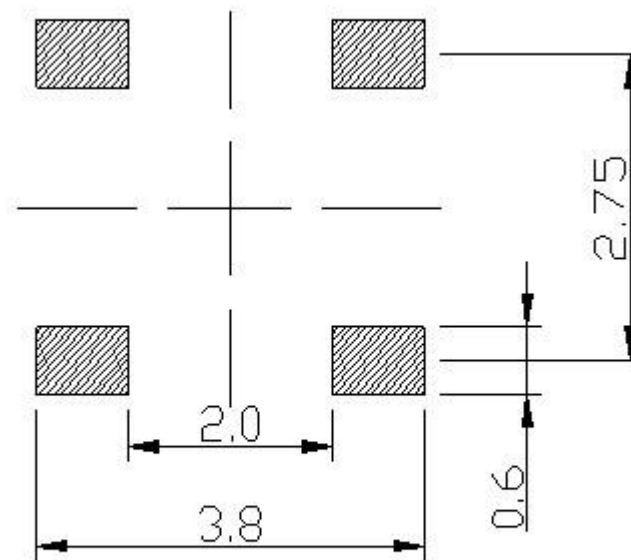
P.C.B LAND DIMENSION
