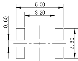
印刷电路板安装孔以及焊接处尺寸图 / PC board mounting hole and land dimensions
