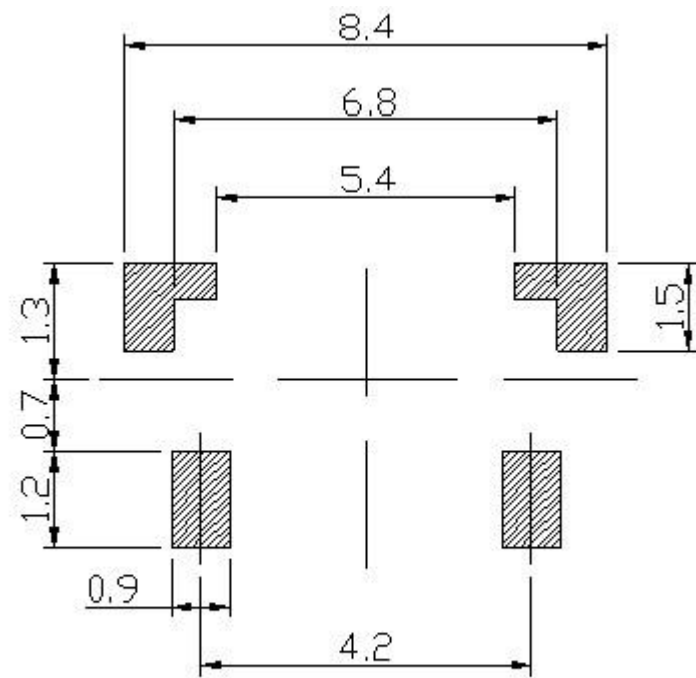
P.C.B LAND DIMENSION
