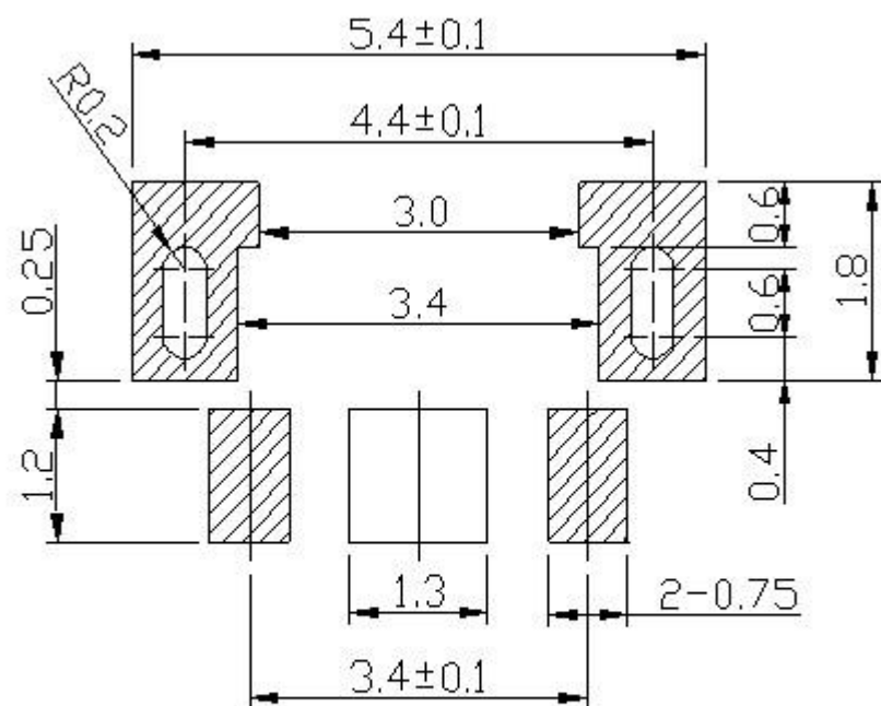
P.C.B LAND DIMENSION
