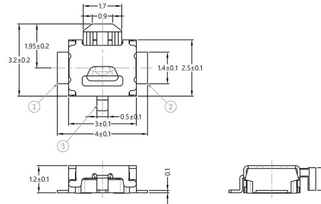
尺寸图 / Dimension Drawing
