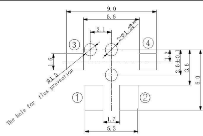
印刷电路板安装孔以及焊接处尺寸图 / PC board mounting hole and land dimensions
